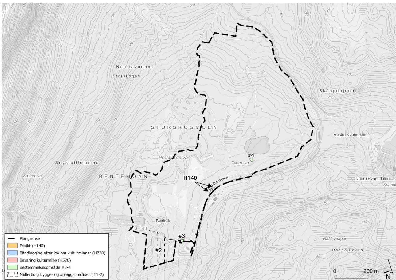
Figur 12: Midlertidige bygge- og anleggsområde, bestemmelsesområder og frisiktsoner på Skoglund.
