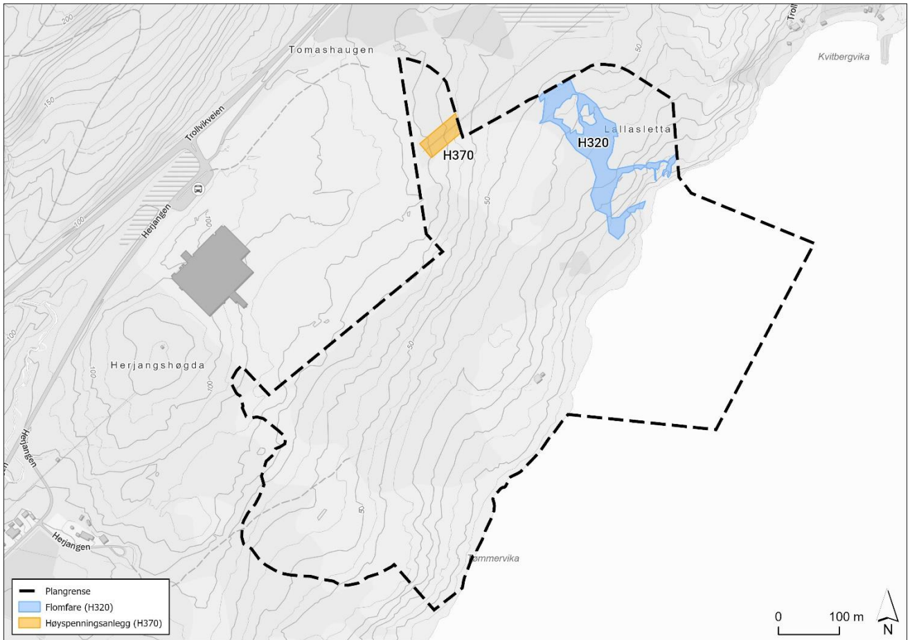
Figur 9: Faresoner for flom og høyspenning på Lallasletta.
