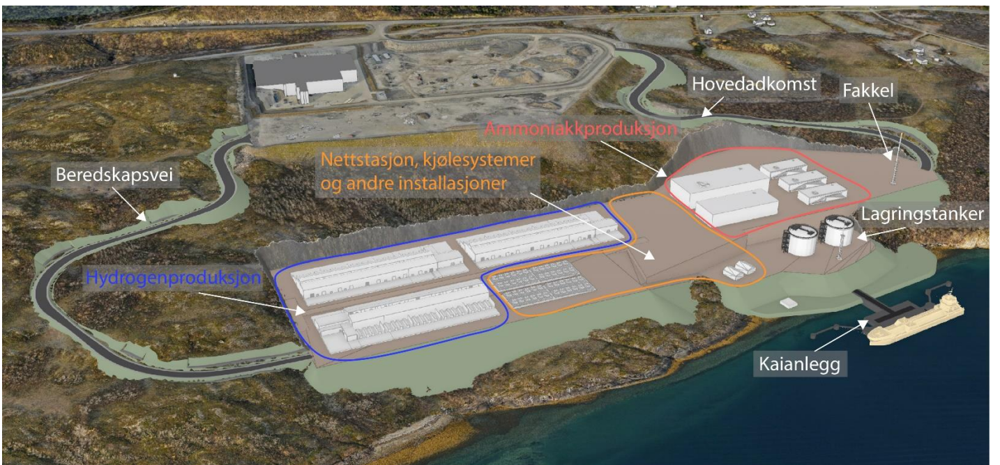
Figur 4: Foreløpig layout for industrianlegg på Lallasletta. Plassering av prosessanleggene internt på tomten er ikke endelig avklart.
