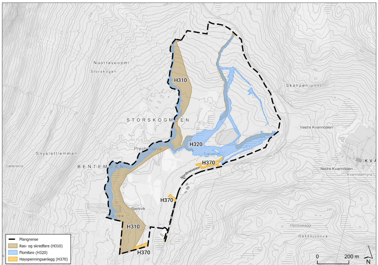
Figur 10: Faresoner for flom, høyspenning, ras og skred på Skoglund.
