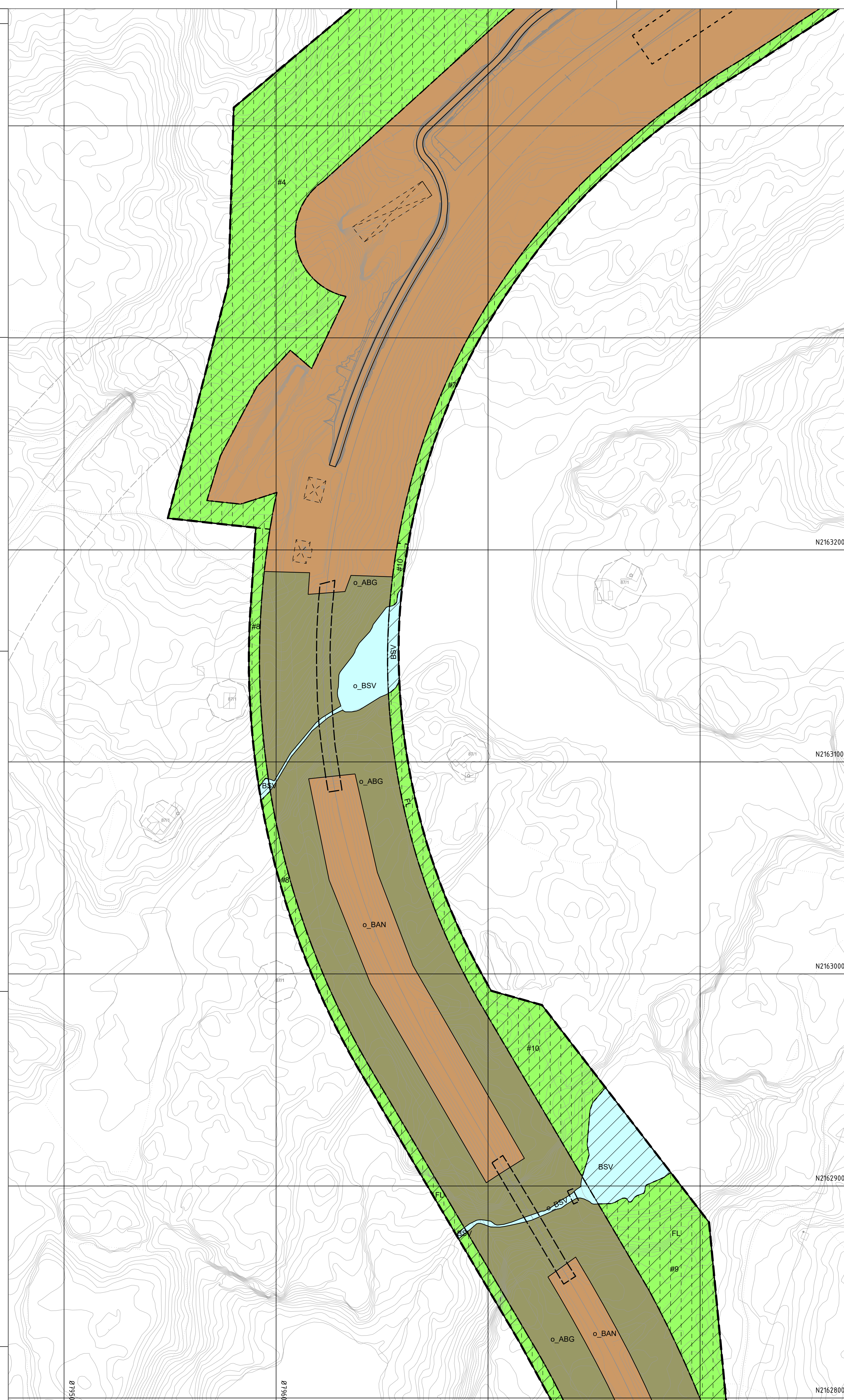
Vertikalnivå 3 - over bakken - Jernbanebru Målestokk: 1:1000
