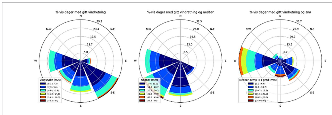
Figur 12: Vindroser for planområdet. Kilde: Streamlit.
