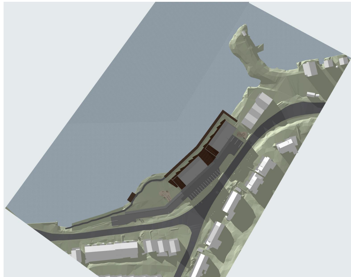
Solstudie 21. juni 22:00
