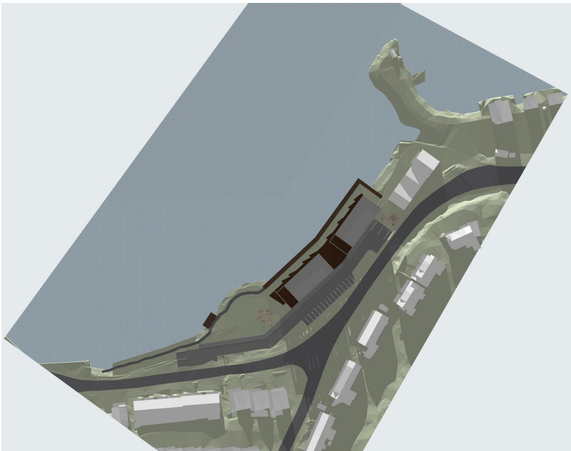
Solstudie 21. juni 00:00
