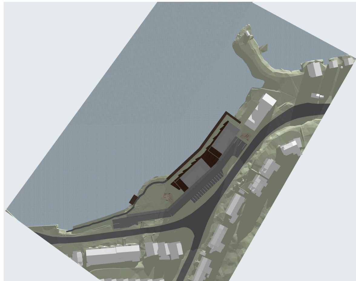
Solstudie 21. juni 02:00
