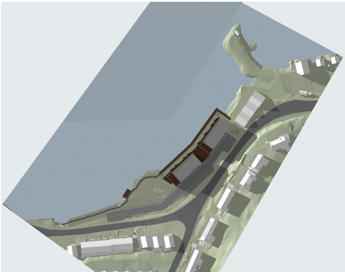
Solstudie 21. juni 20:00
